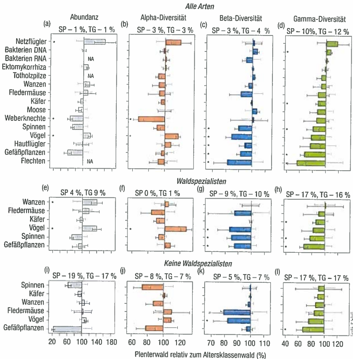
Abb. 3: Abundanz, Alpha-, Beta- und Gamma-Diversität (jeweils OD) der 15 untersuchten Artengruppen von Altersklassenwald und Plenterwald im Vergleich. Die Skala auf der x-Achse zeigt die Richtung der Unterschiede an. Säulen, die nach links zeigen (Werte < 100), weisen auf geringere, Säulen, die nach rechts zeigen (Werte > 100), auf höhere Werte im Plenterwald hin. Signifikante Unterschiede sind durch ein Sternchen gekennzeichnet. Dargestellt sind die Ergebnisse für alle Arten (a-d) und für diejenigen Artengruppen, für die Waldartenlisten vorliegen. Für diese erfolgte eine getrennte Darstellung nach Waldspezialisten (e-h) und Nicht-Waldspezialisten (i-l). Verändert aus [10]. TG -12 % bedeutet, dass über alle Artengruppen hinweg im Plenterwald 12 % weniger Arten vorhanden sind als im Altersklassenwald; bei SP werden bei der Mittelbildung die Artengruppen entsprechend ihrer Artenzahl gewichtet.
